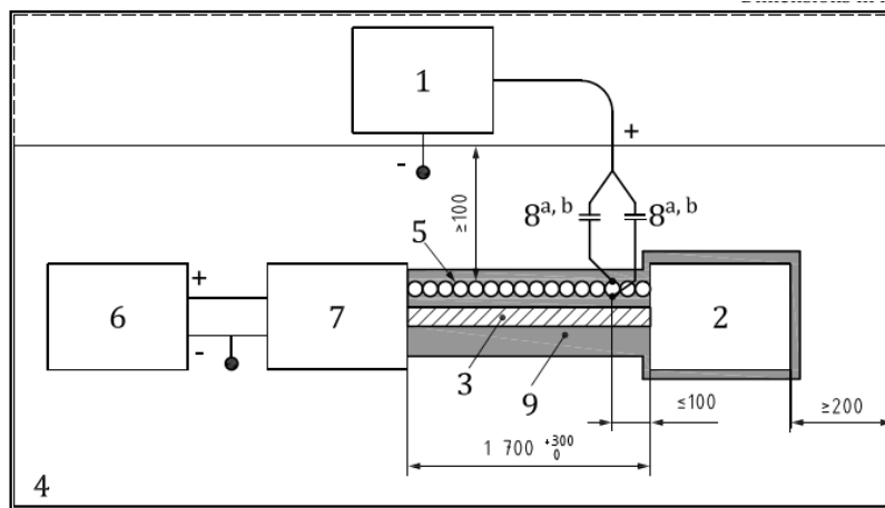
图4 DCC 法试验布置
