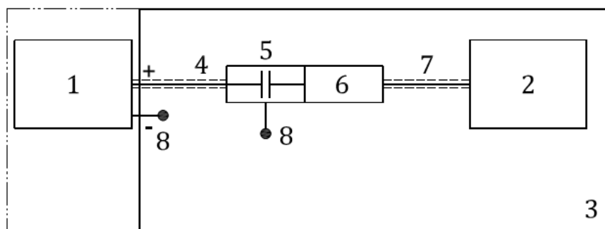
a) 慢速瞬态脉冲
