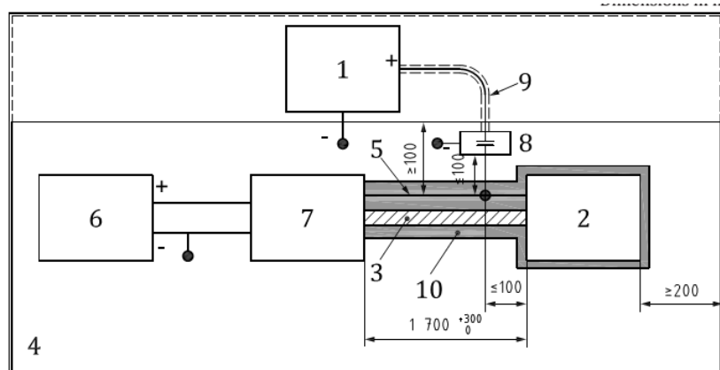
a) 慢速瞬态脉冲试验
