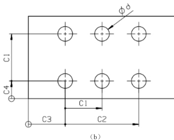
图 1 组孔内中心距和孔边距
