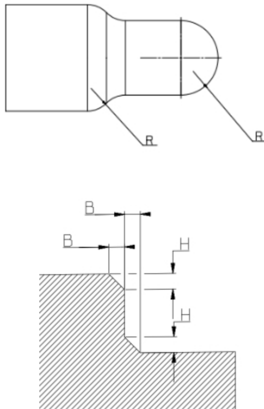
图 3 未注倒角和圆角半径
