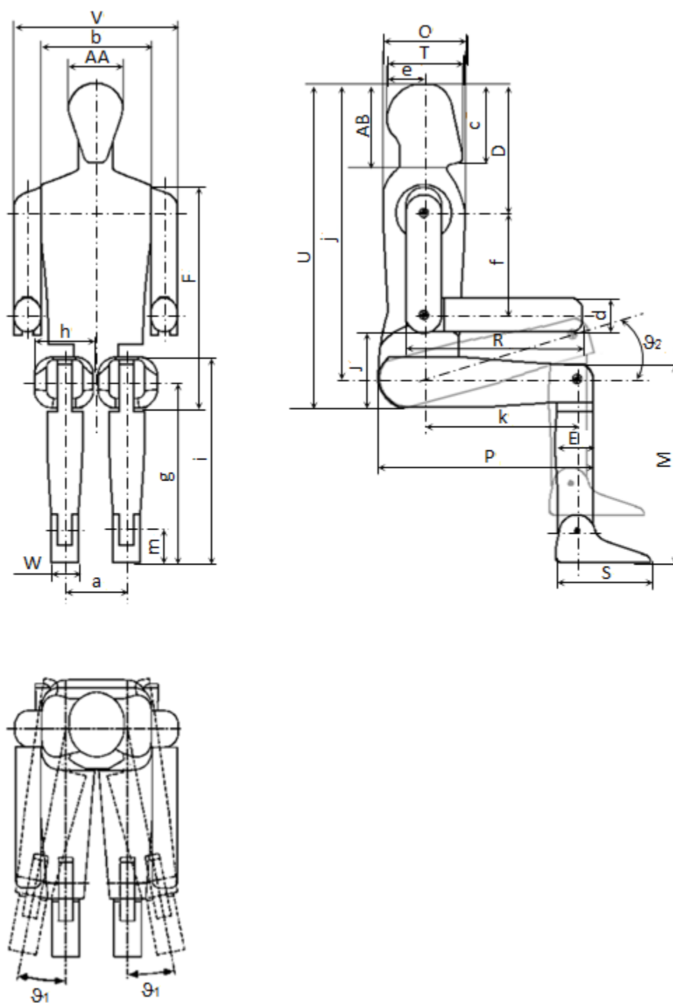
图 B.1 人体模型
