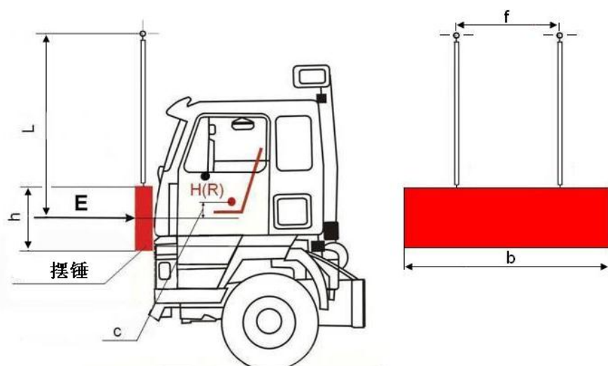
图1 正面撞击试验（试验A）
