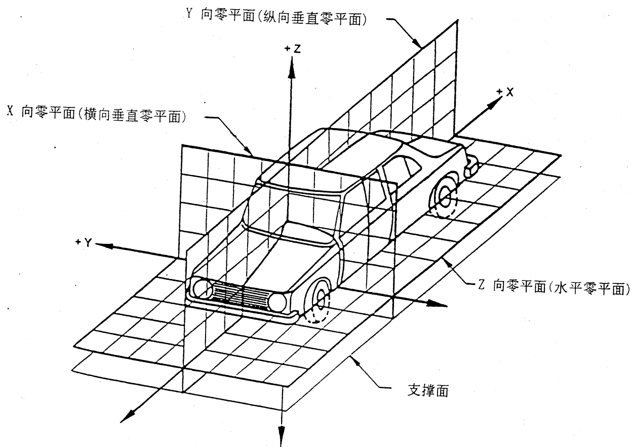
图 C.1 三维坐标系
