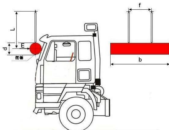
图2 A柱撞击试验（试验B）
