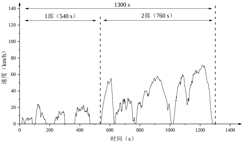
图 错误！文档中没有指定样式的文字。 CHTC-D行驶工况
