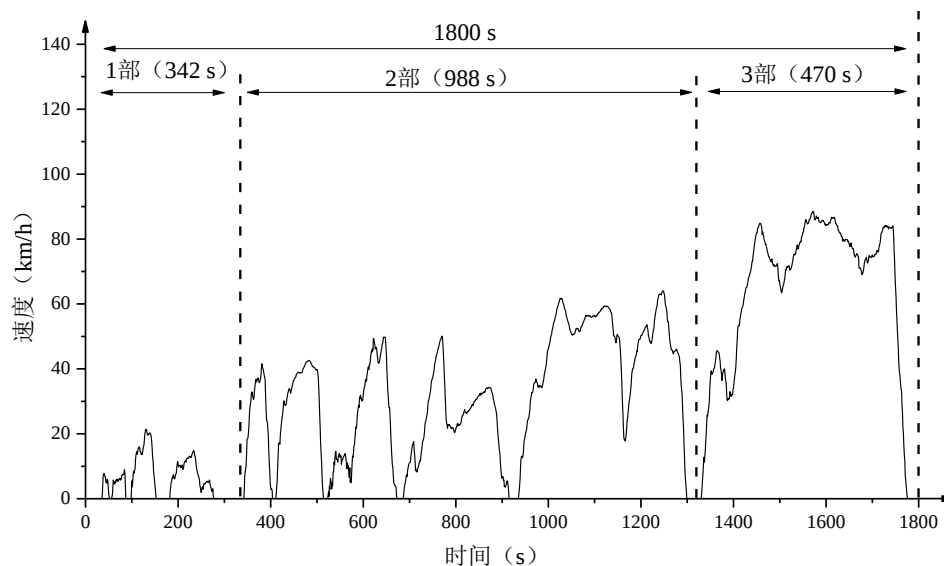
图3 CHTC-HT行驶工况
