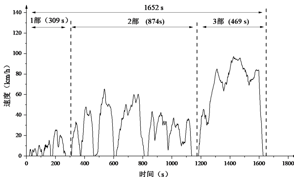
图4 CHTC-LT行驶工况
