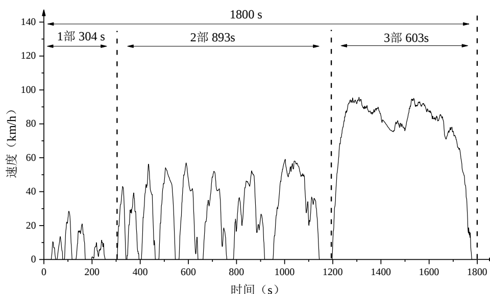
图2 CHTC-C行驶工况
