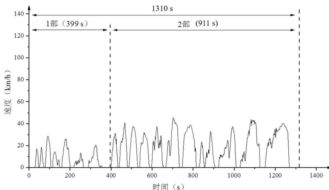
图1 CHTC-B行驶工况
